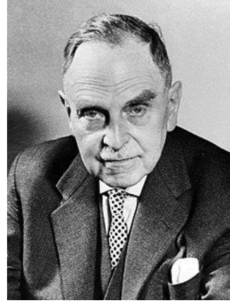
اوتو هان
