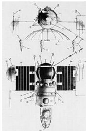
ونرا ۷
