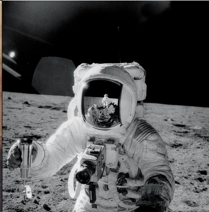
آپولو ۱۲
